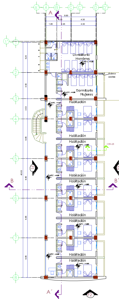
PLANTA ALTA
