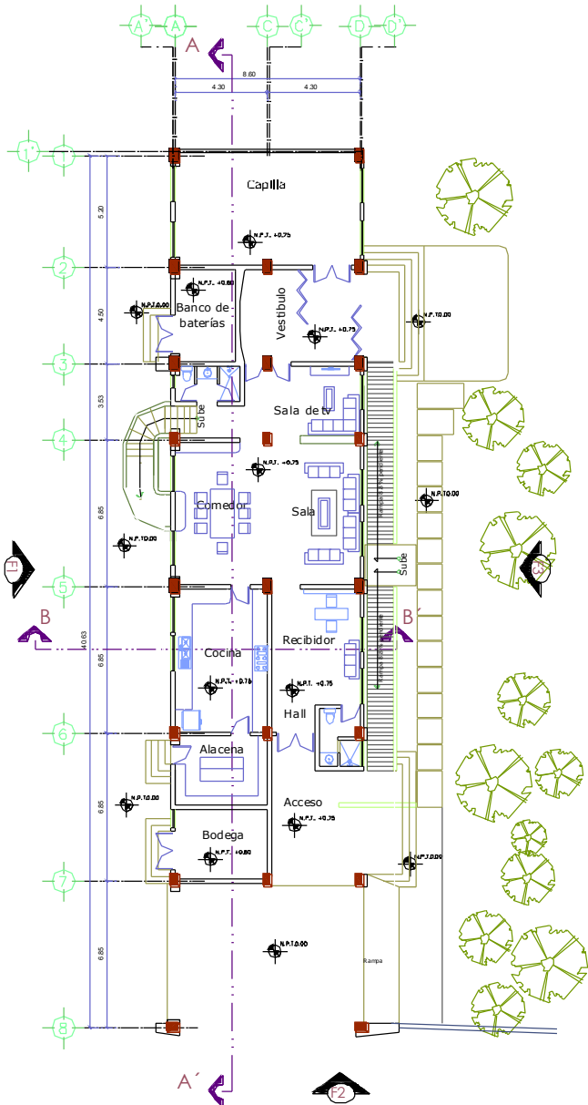
PLANTA BAJA
